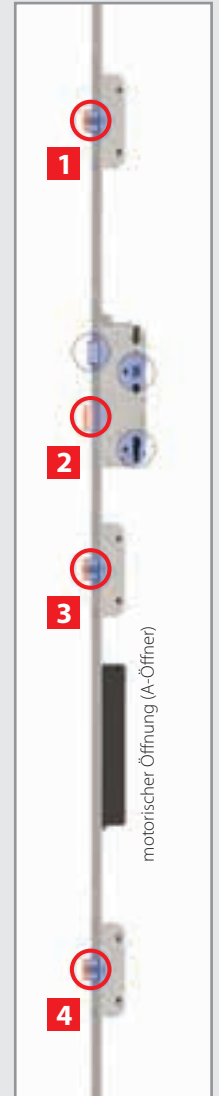
4-fach Verriegelung Automatik GU SECURITY A3 mit motorischer Öffnung (A-Öffner)
