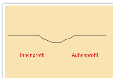
◀ Querschnitt Profil Profundo
